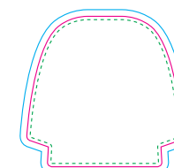
シールサイズ (ピンク線) 23.3×22.5mm
